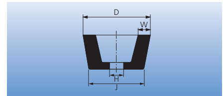
Cup wheel ETT
